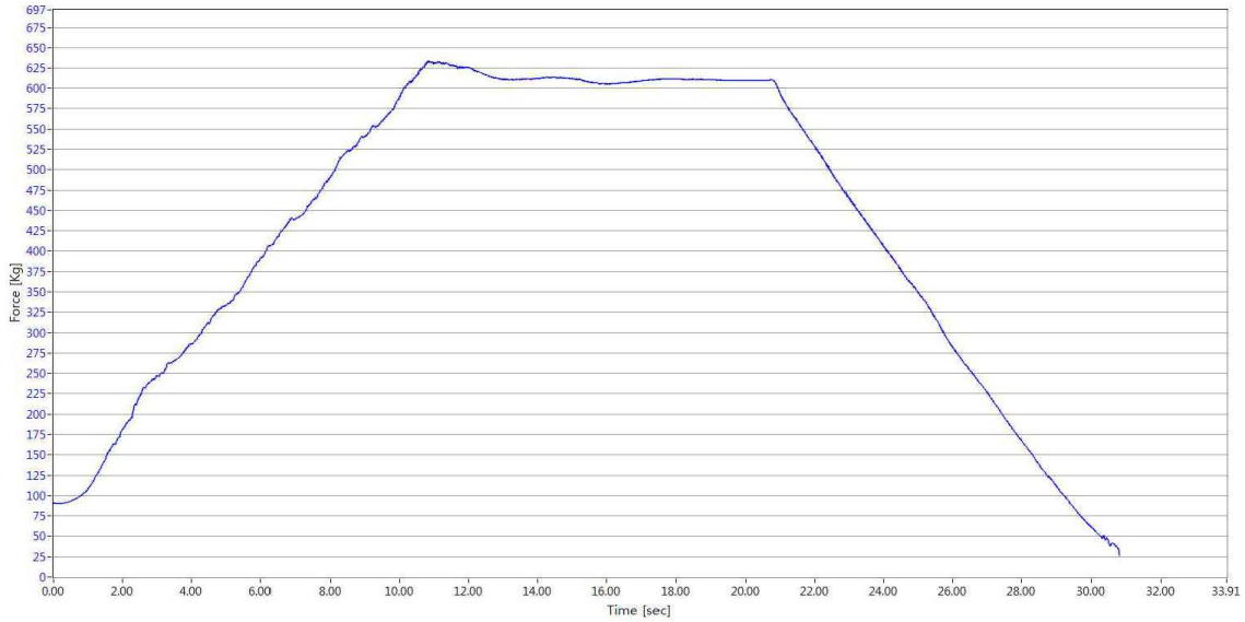
<그림 3> 서원시트 카니발KA4 3열 LH,RH 연결 좌석 강도시험 시간-하중 그래프
