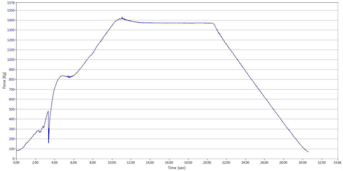
<그림 8> 서원시트 카니발KA4 3열(연결) LH 어깨 좌석안전띠부착장치 강도시험 시간-하중 그래프
