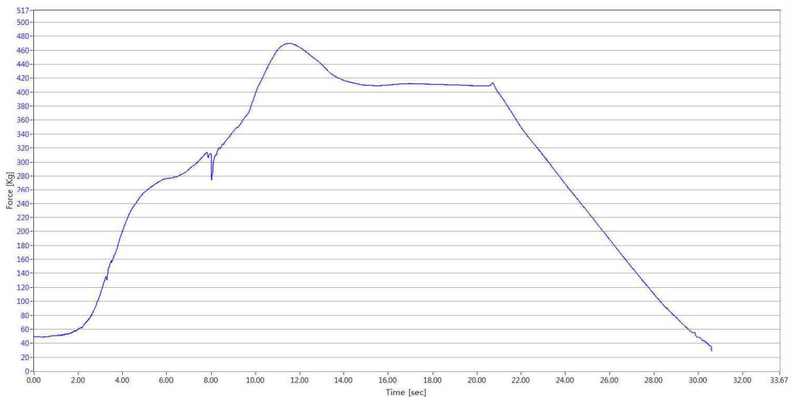
<그림 2> 서원시트 카니발KA4 3열 LH 좌석 강도시험 시간-하중 그래프
