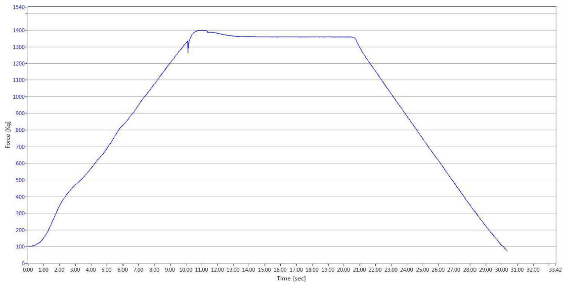
<그림 7> 서원시트 카니발KA4 3열 LH 골반 좌석안전띠부착장치 강도시험 시간-하중 그래프
