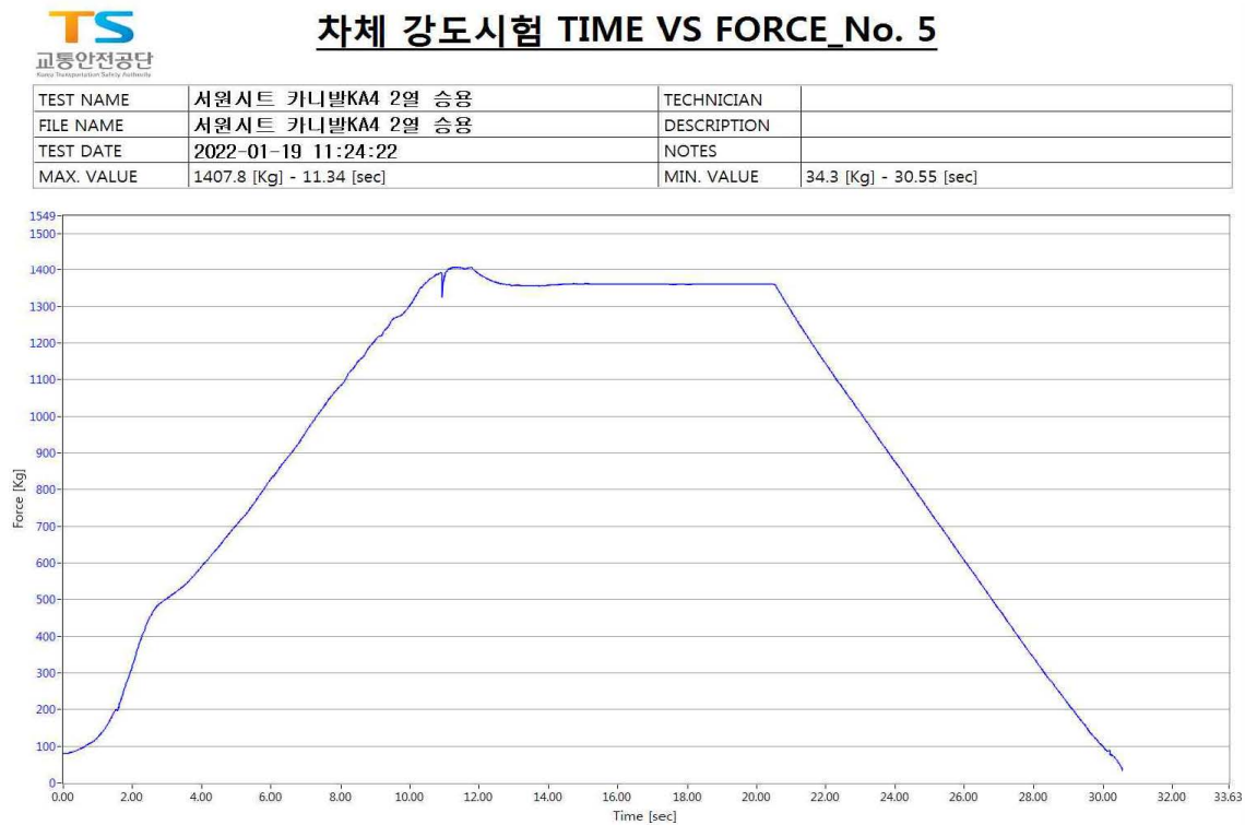
<그림 5> 서원시트 카니발KA4 2열 RH 골반 좌석안전띠부착장치 강도시험 시간-하중 그래프
