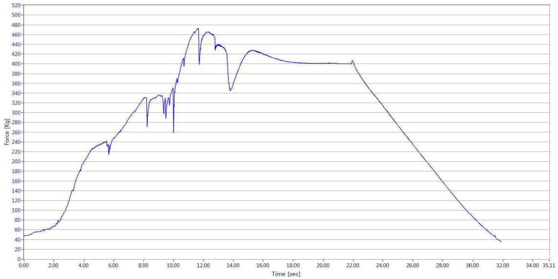
<그림 1> 서원시트 카니발KA4 2열 RH 좌석 강도시험 시간-하중 그래프
