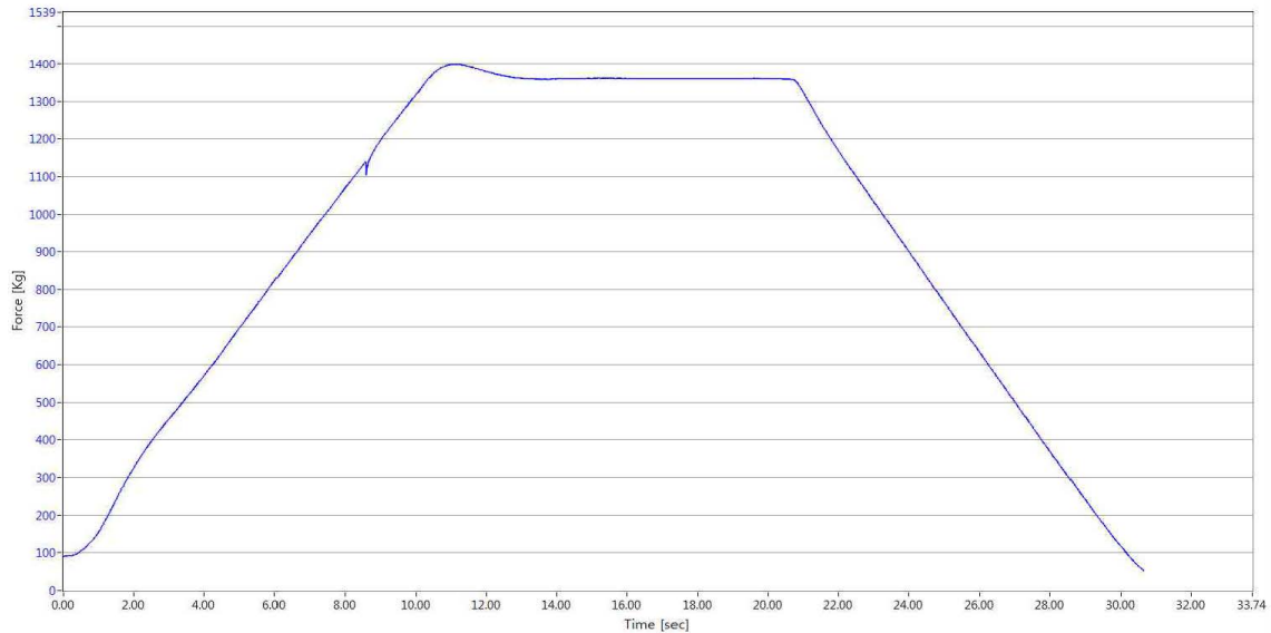
<그림 6> 서원시트 카니발KA4 3열 LH 어깨 좌석안전띠부착장치 강도시험 시간-하중 그래프
