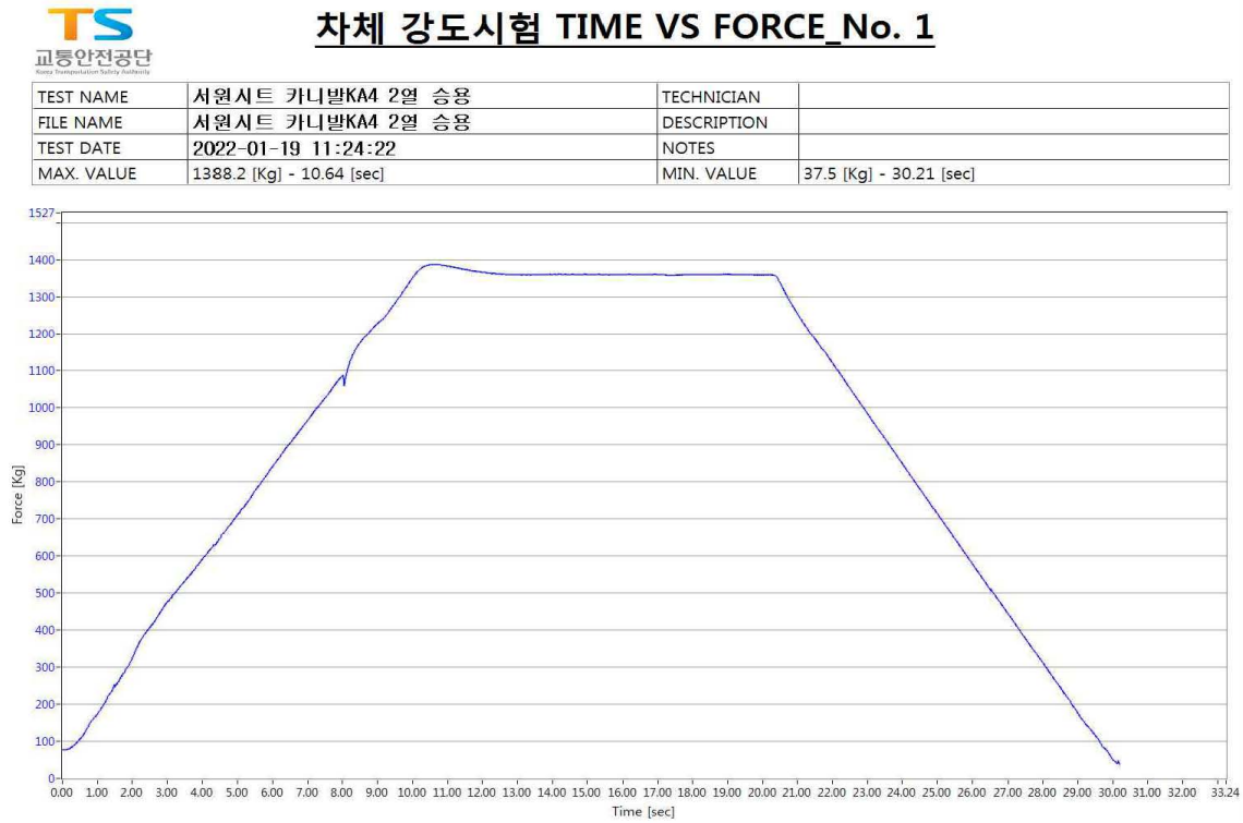
<그림 4> 서원시트 카니발KA4 2열 RH 어깨 좌석안전띠부착장치 강도시험 시간-하중 그래프
