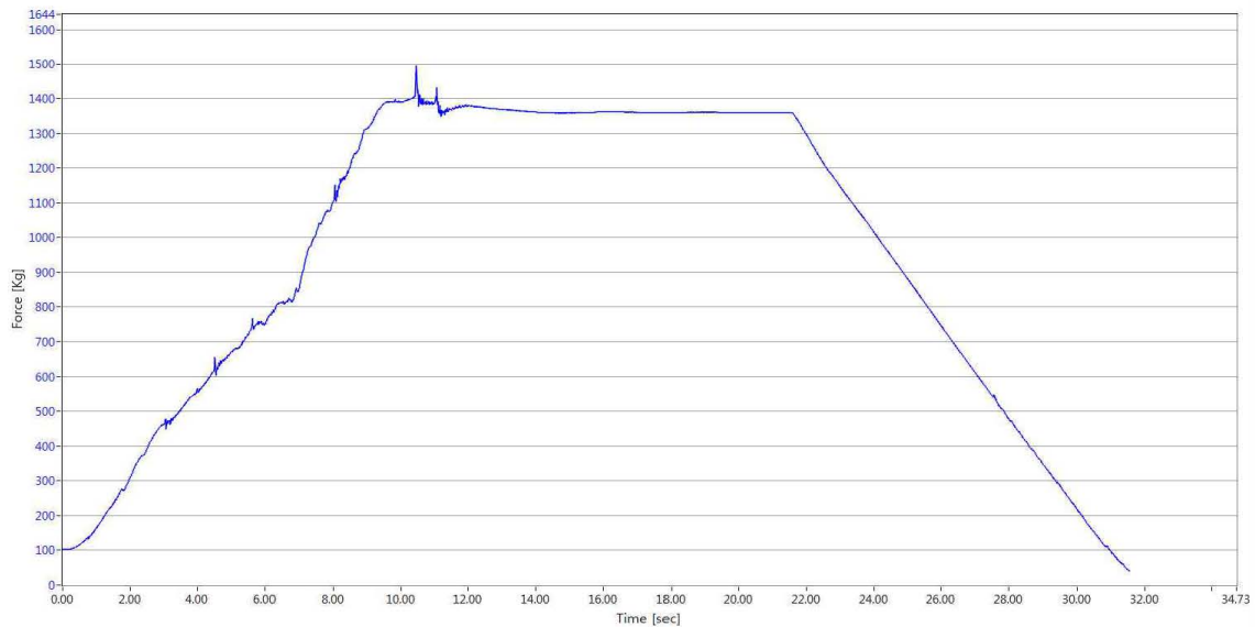
<그림 10> 서원시트 카니발KA4 3열 연결 RH 어깨 좌석안전띠부착장치 강도시험 시간-하중 그래프
