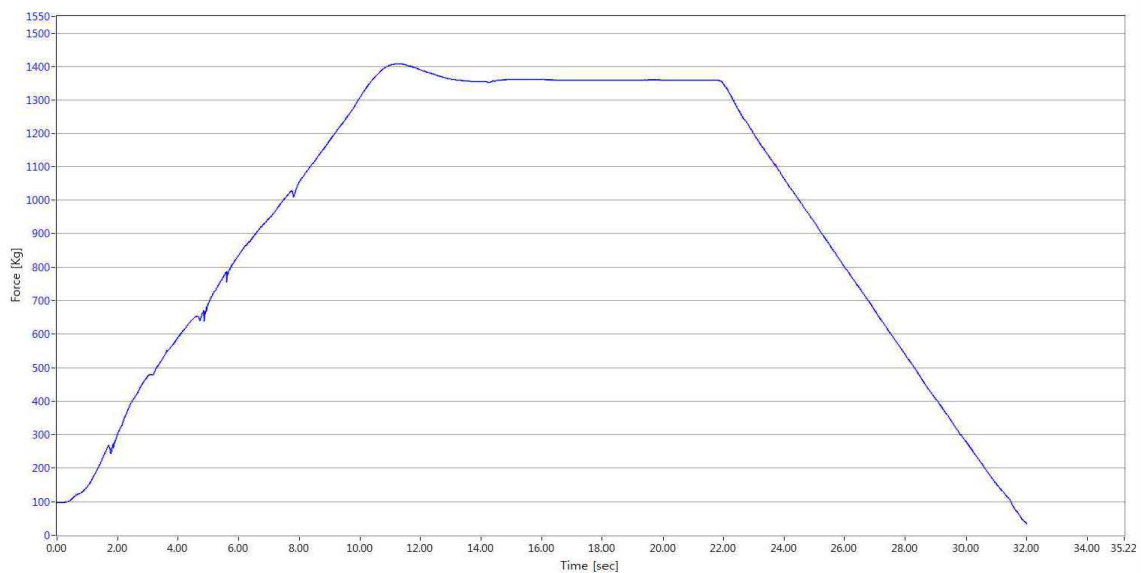
<그림 11> 서원시트 카니발KA4 3열 연결 RH 골반 좌석안전띠부착장치 강도시험 시간-하중 그래프
