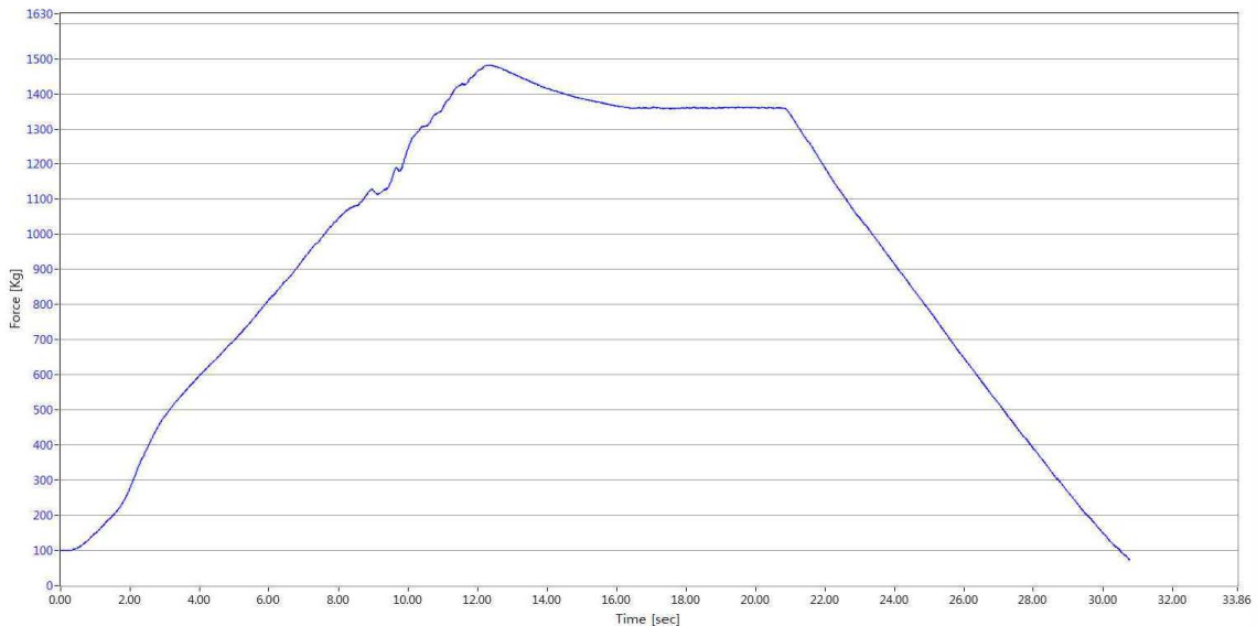
<그림 9> 서원시트 카니발KA4 3열(연결) LH 골반 좌석안전띠부착장치 강도시험 시간-하중 그래프
